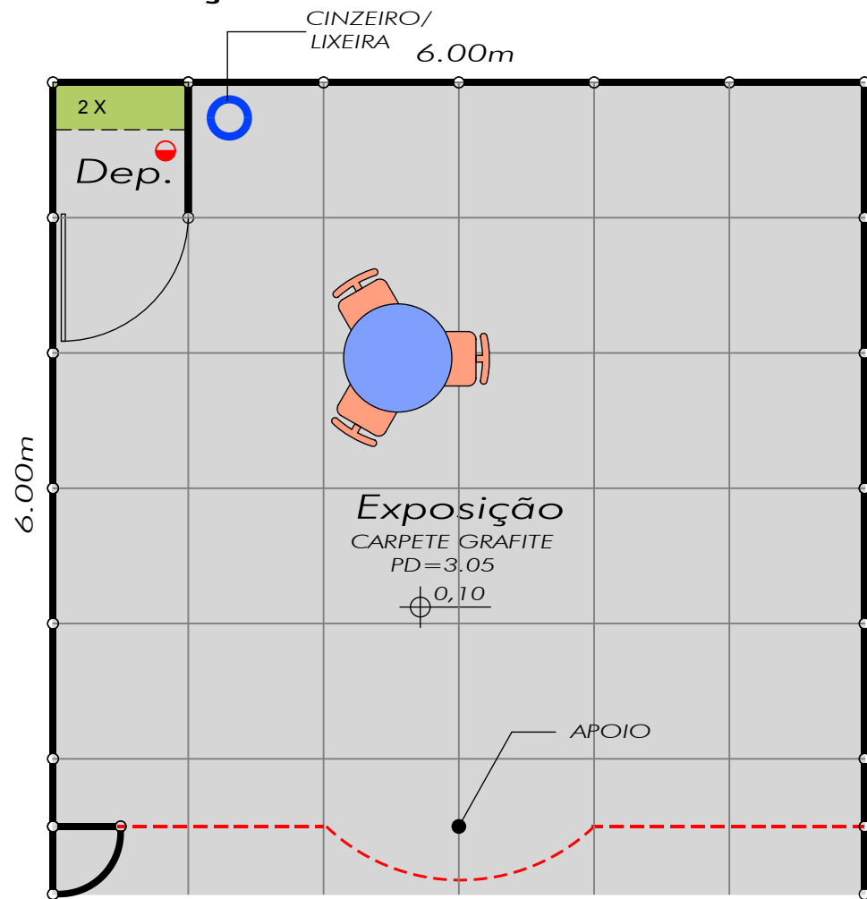
PLANTA ESC. 1/50
